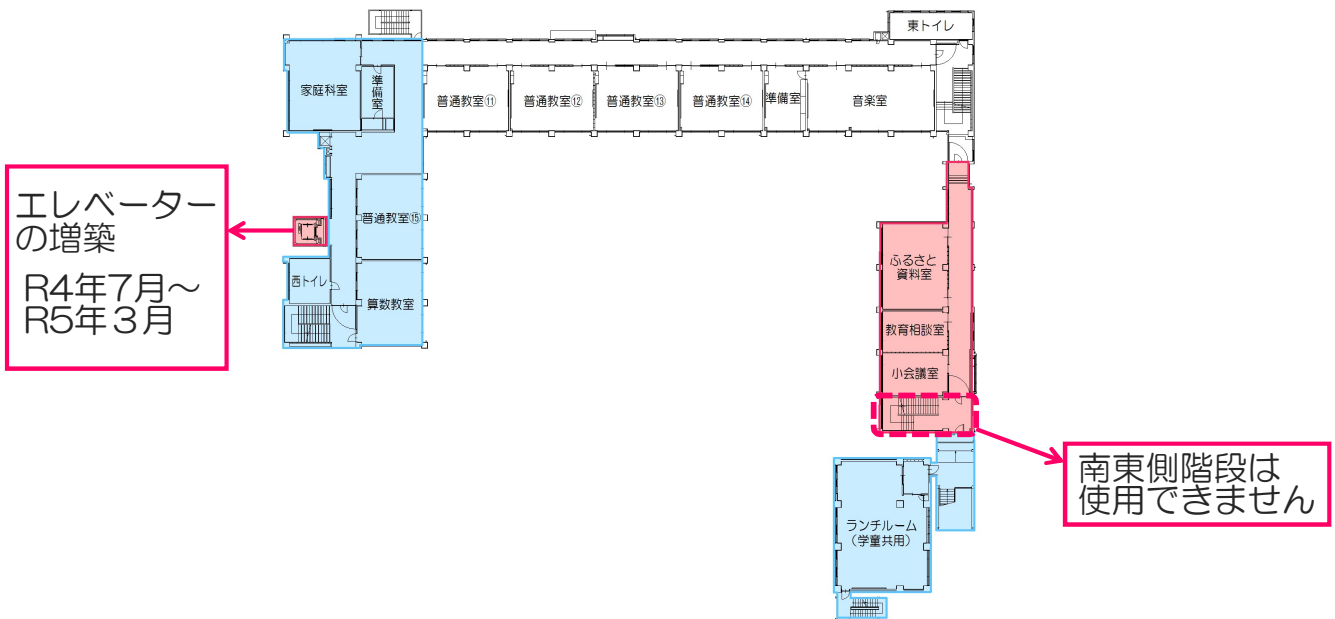
3階平面図
