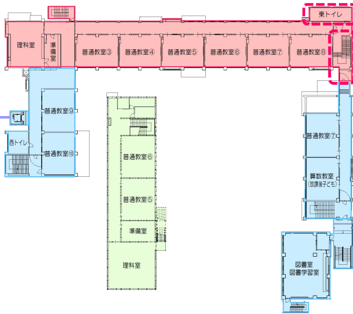
2階平面図
