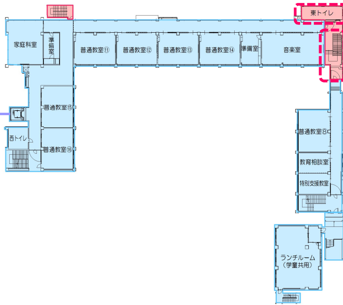
3階平面図
