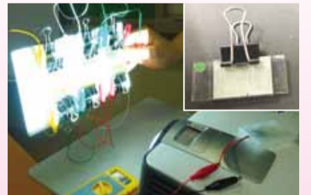
色素増感型太陽電池を直列につなげて発電しているところ
